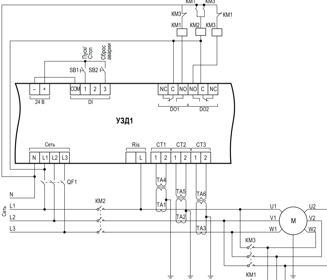
Рисунок 4.1 – Электрическая схема реализации реверсивного режима работы электродвигателя**
