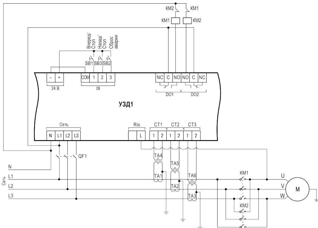
Рисунок 4.1 – Электрическая схема реализации реверсивного режима работы электродвигателя**
