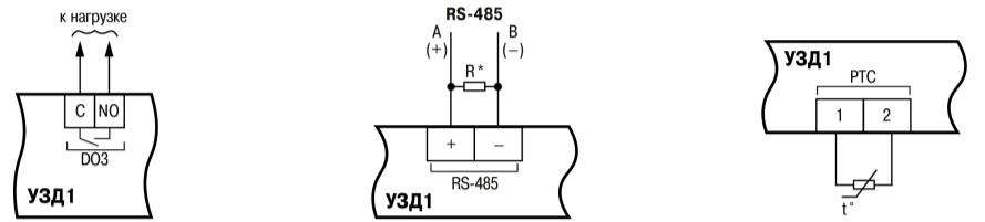
Рисунок 4.5 – Схема подключения DO3
