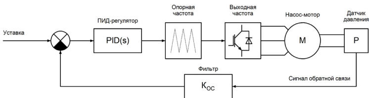
Рисунок 6.16 – Схема ПИД-регулирования
