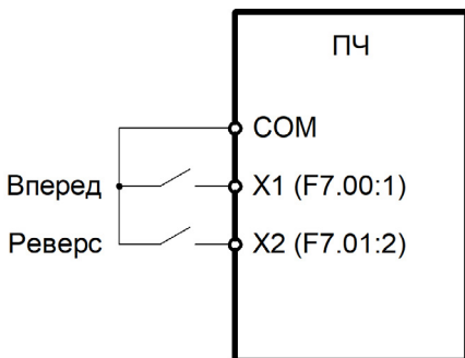
Рисунок 6.12 – Схема двухпроводного подключения 1
