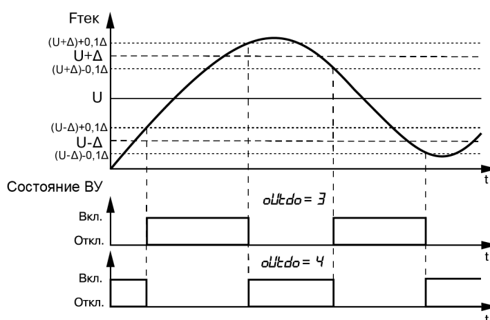
Рисунок 7.7 – Типы логики (П- и U-образная) при работе ВУ в качестве компаратора
