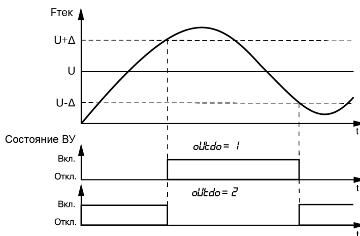
Рисунок 7.6 – Типы логики (обратный и прямой гистерезис) при работе ВУ в качестве компаратора
