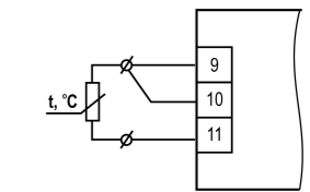
Рисунок 7 – Подключение ТС по трехпроводной схеме
