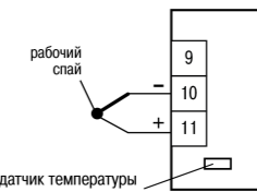
Рисунок 6 – Схема подключения ТП
