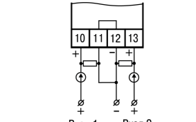
Рисунок 9 – Подключение активных датчиков
