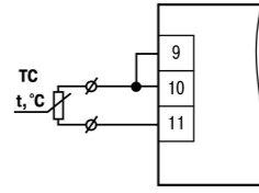
Рисунок 8 – Подключение ТС по двухпроводной схеме
