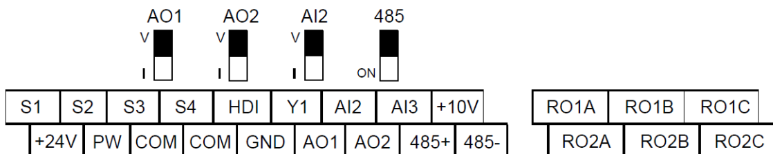
Рис. 5-18 Клеммы цепей управления приводов 4 кВт и более
